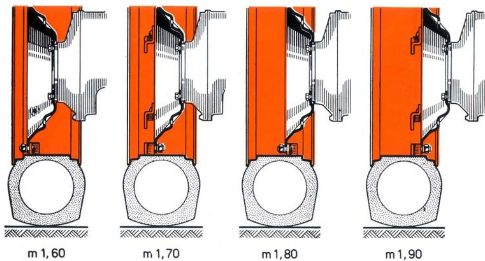
FIG. 12. — Variation de la voie arrière.
