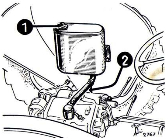
FIG. 42 — Réservoir auxiliaire.
