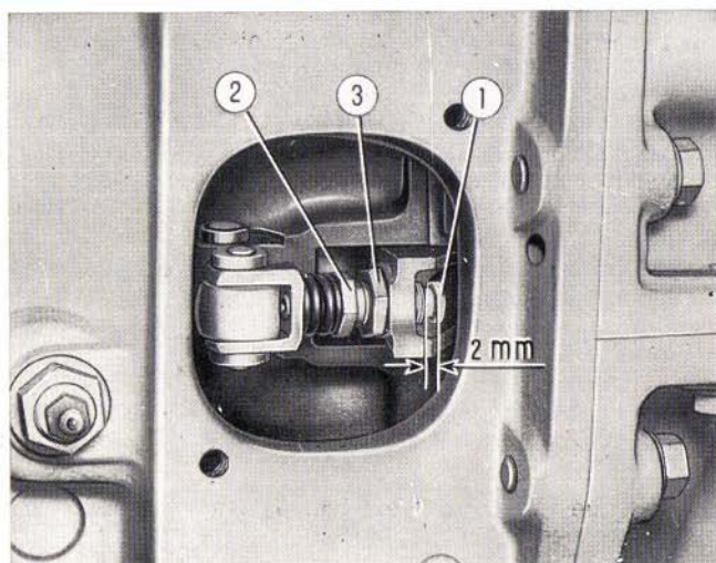
FIG. 25 — Réglage des tirants de débrayage de la prise de force 1. Tirant - 2. Vis de réglage du jeu - 3. Ecrou de blocage de la vis.
