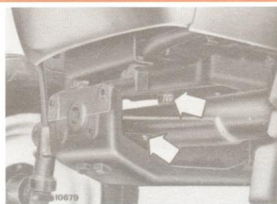
15 AXE D'ARTICULATION D'ESSIEU ET AXE DE RENVOI DIRECTION - Injecter de la graisse FIAT G 9 avec la pompe dans les 2 graisseurs.
