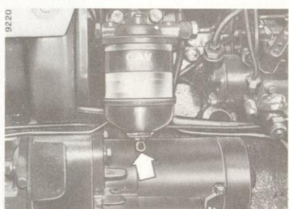
13 PREMIER FILTRE A COMBUSTIBLE - Vidanger l'eau en desserrant de 3-4 tours la vis inférieure et en manoeuvrant le levier de pompe d'alim.
