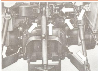
9 RELEVAGE ET DISPOSITIF D'ATTELAGE OUTILS - Injecter de la graisse FIAT G 9 avec la pompe (6 graisseurs).
