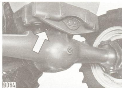
16 AXE DE PIVOITEMENT DE PONT AV (DT) - Injecter de la graisse FIAT G 9 avec la pompe.
