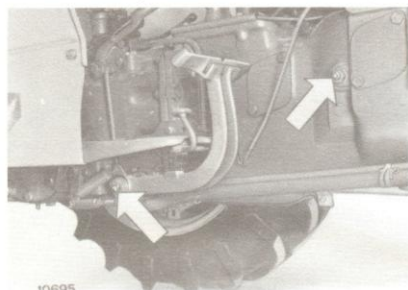
11 EMBRAYAGE ET ARBRE DE PEDALES - Injecter de grassofiat G 9 (3 graisseurs, 1 par côté sur l'arbre). Deux coups dans le graisseur d'embrayage.
