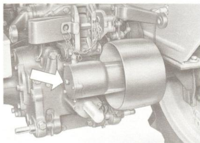
10 POULIE MOTRICE - Vérifier que l'huile arrive au bouchon; faire l'appoint, si nécessaire, par ce même bouchon (huile FIAT AMBRA 20W/40).
