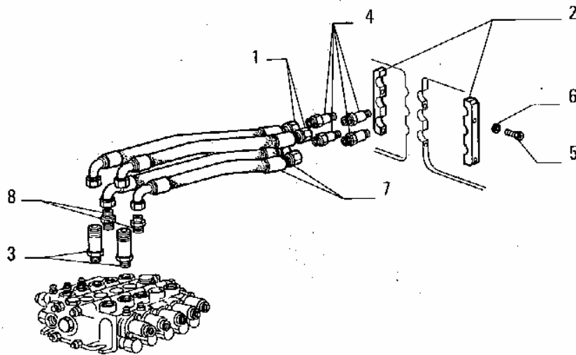
BACK-HOE RETRDESCAVATORE
