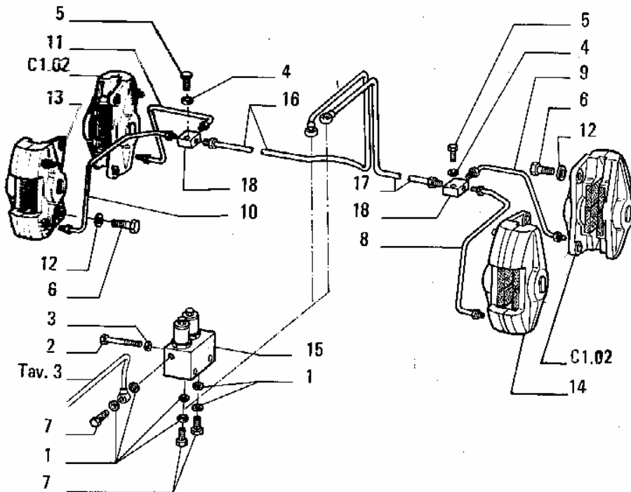
CALIPER PINZA FRENO
