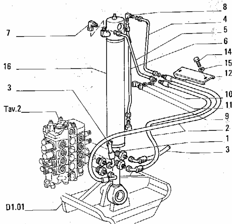
STABILIZER CYLINDER CILINDRO STABILIZZATORE
