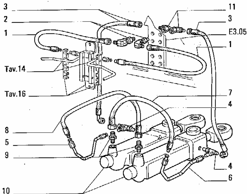
BACK HOE SWING CYLINDER CILINDRO ROTAZIONE RETRO
