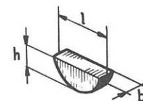
CLAVETTE DISQUE
