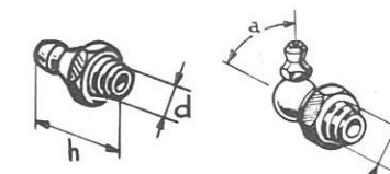
GRAISSEUR " HYDRAULIC "
