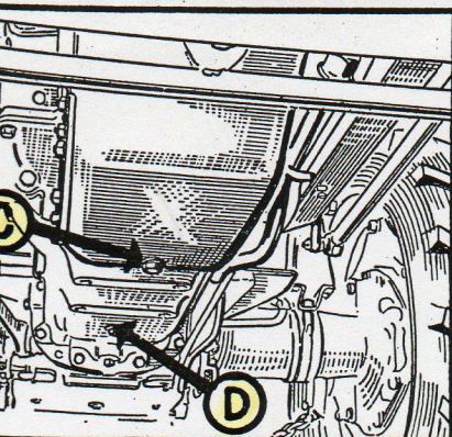
CARTER D'HUILE MOTEUR - Vidanger par C. Evacuer les dépôts dans le carter d'embrayage par D.
