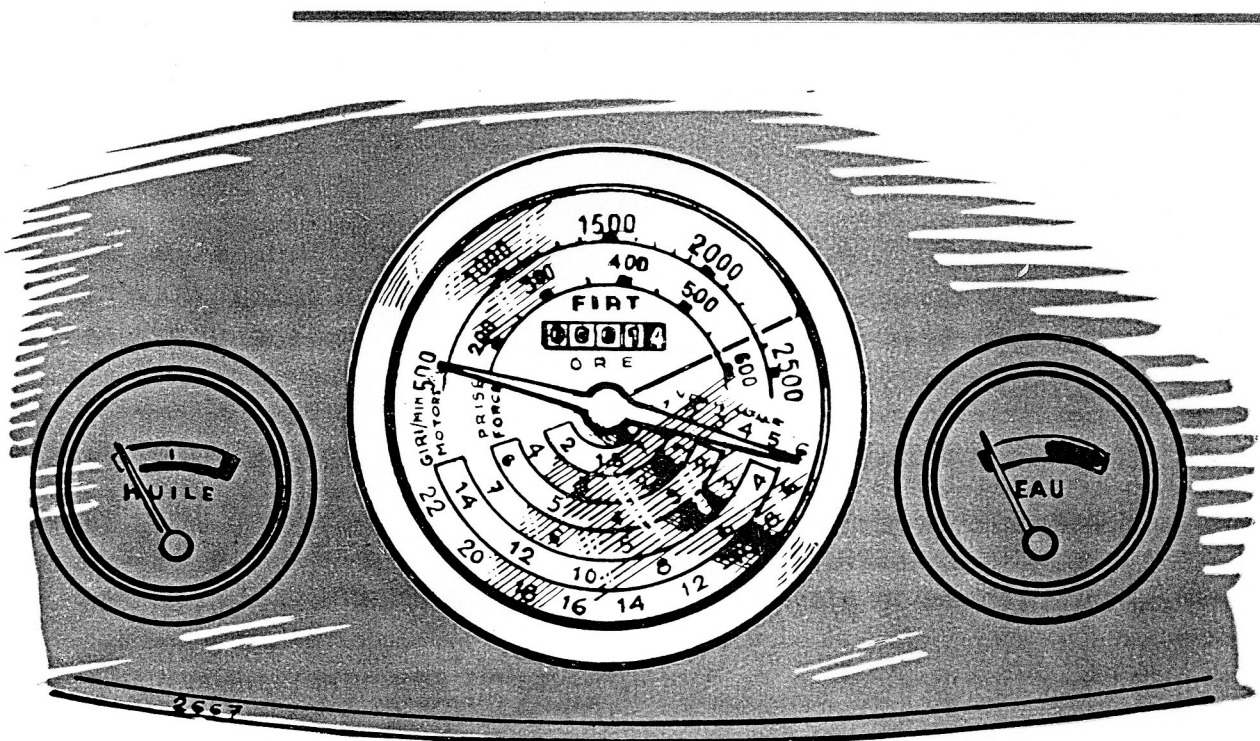
FIG. 18 — Horomètre. Au centre de l'horotachymètre.
