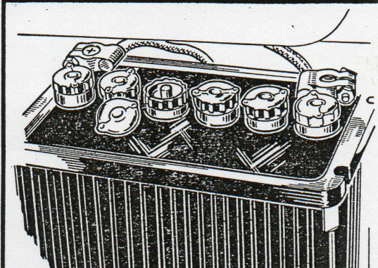
21 BATTERIES - Parfaire le ni- veau avec de l'eau distillée. (1 cm au-dessus des plaques).
