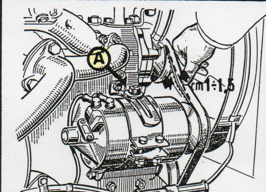
17 COURROIE DE VENTILA- TEUR ET DYNAMO - Vérifier la tension. A : écrou de tension.
