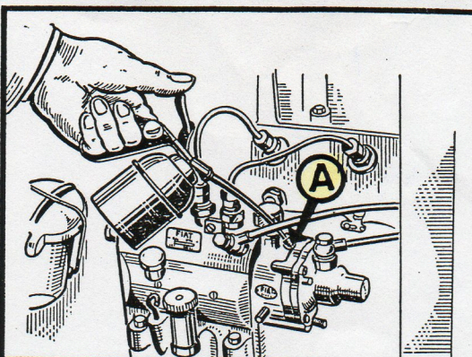
16 REGULATEUR DE VITESSE Introduire deux ou trois gouttes d'huile et pas davan- tage par l'orifice A.
