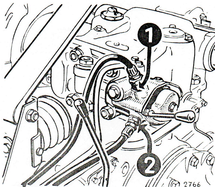
FIG. 37 — Distributeur auxiliaire équipé en double effet.
