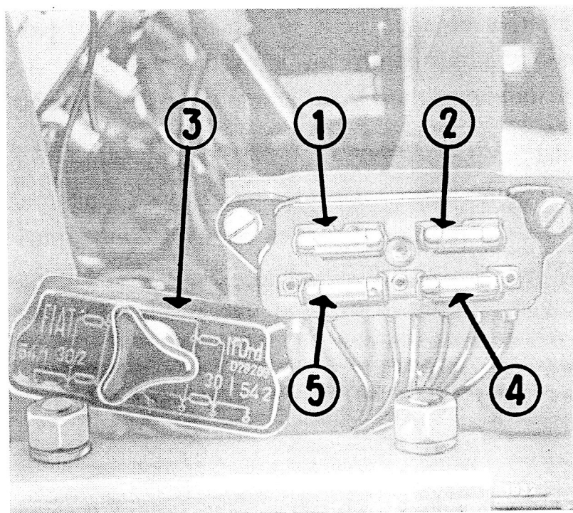
FIG. 25. — Fusibles de protection des appareils d'éclairage.
