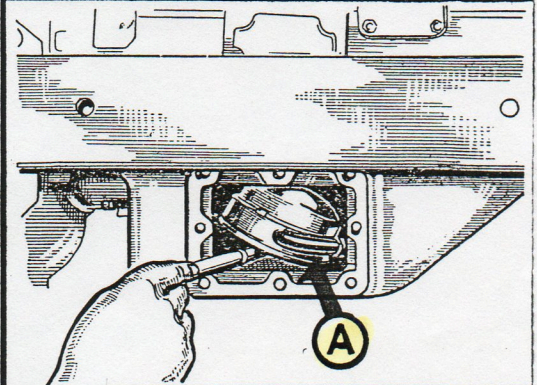
23 FILTRE D'ASPIRATION D'HUILE DU MOTEUR - Après la vidange nettoyer la crépine A au pétrole
