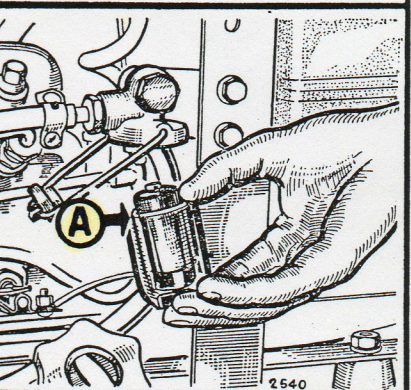
POMPE D'ALIMENTATION Déposer la cuve de décan- tation et laver le filtre au pétrole.
