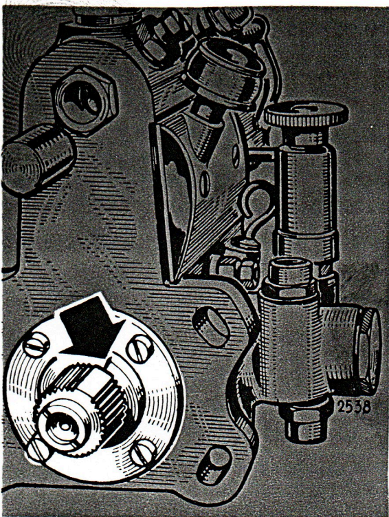
Fig. 30 A. Orientation du pignon pour faciliter la mise en place de la pompe d'injection.
