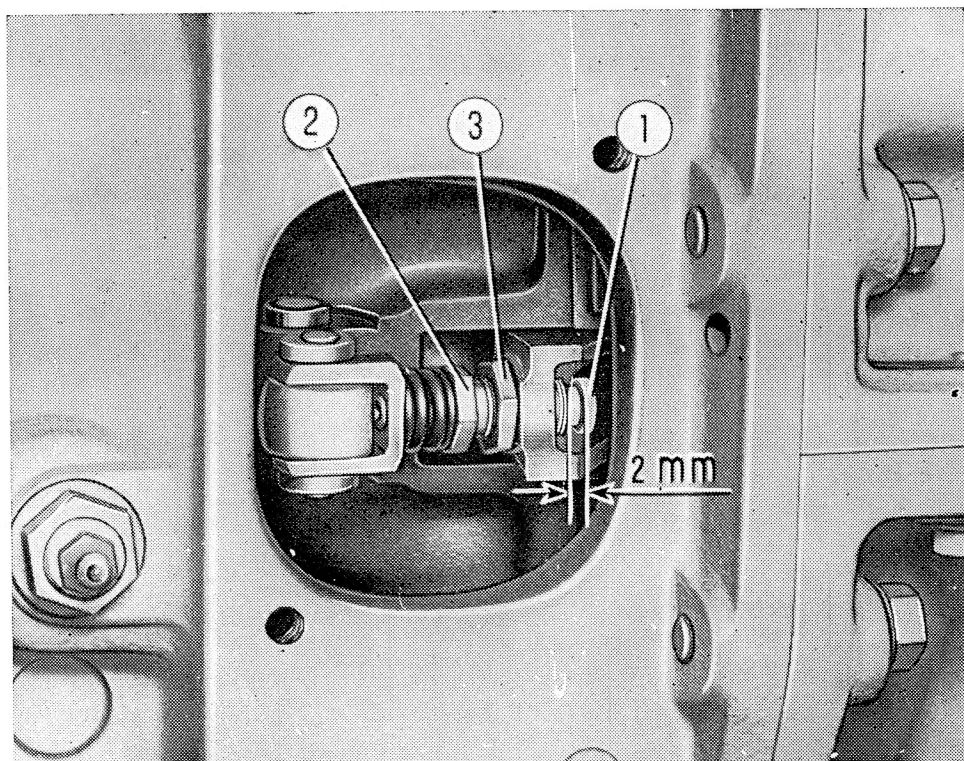
FIG. 21. — Réglage des tirants de débrayage de la prise de force.
