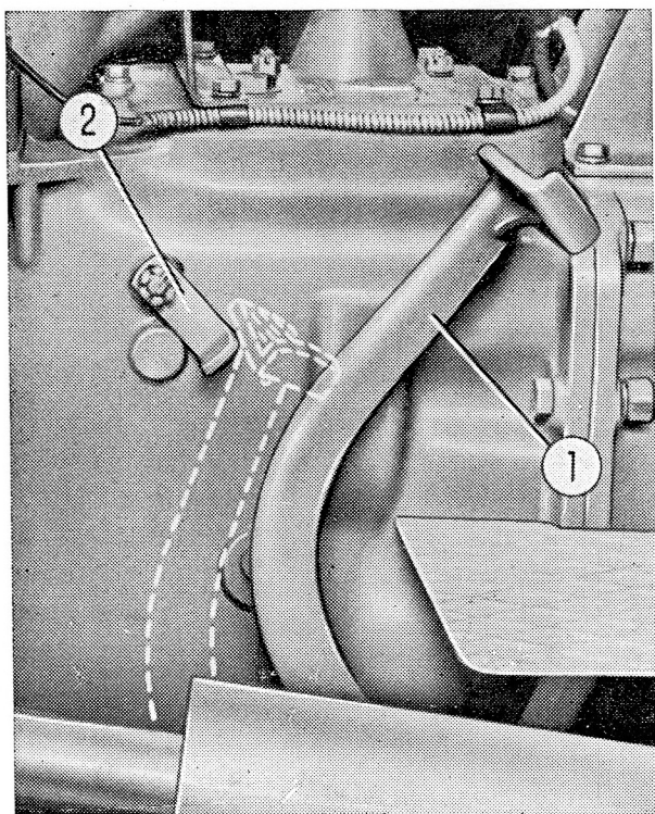
FIG. 6 A. — Pédale de débrayage (1) avec course limitée par la butée (2)
