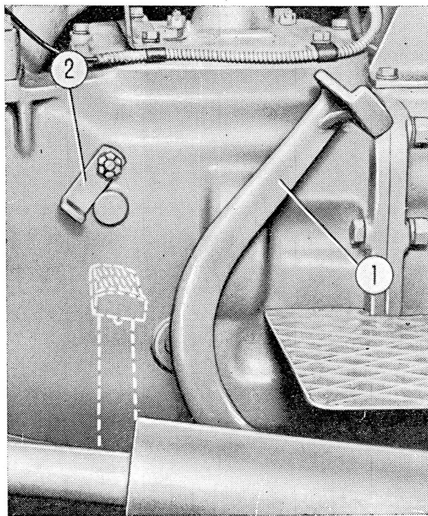
FIG. 6 B. — Pédale de débrayage (1) avec butée (2) libérant la course totale.
