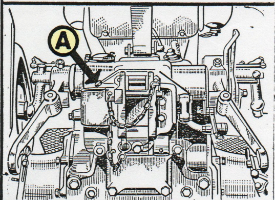
22 RELEVAGE HYDRAULIQUE Vérifier le niveau d'huile. A= niveau et remplissage.
