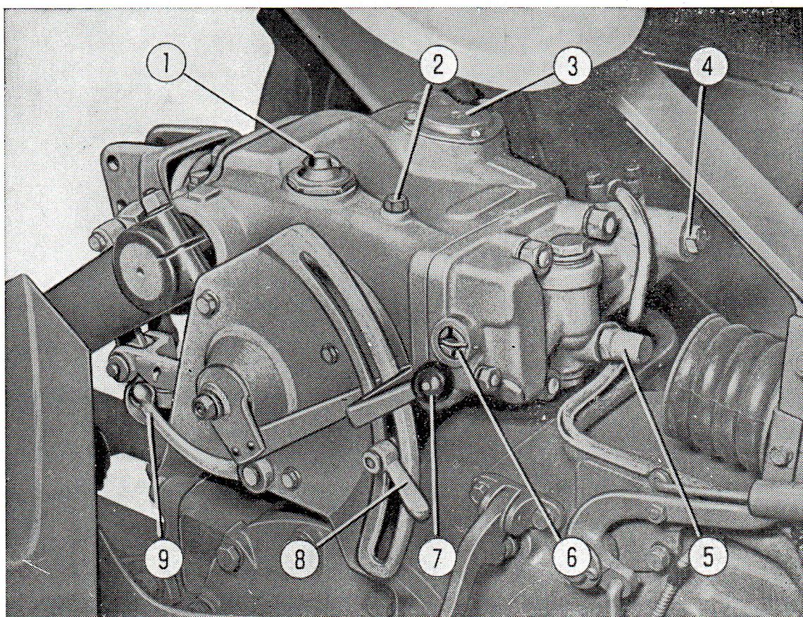
FIG. 12. — Dispositif de relevage
