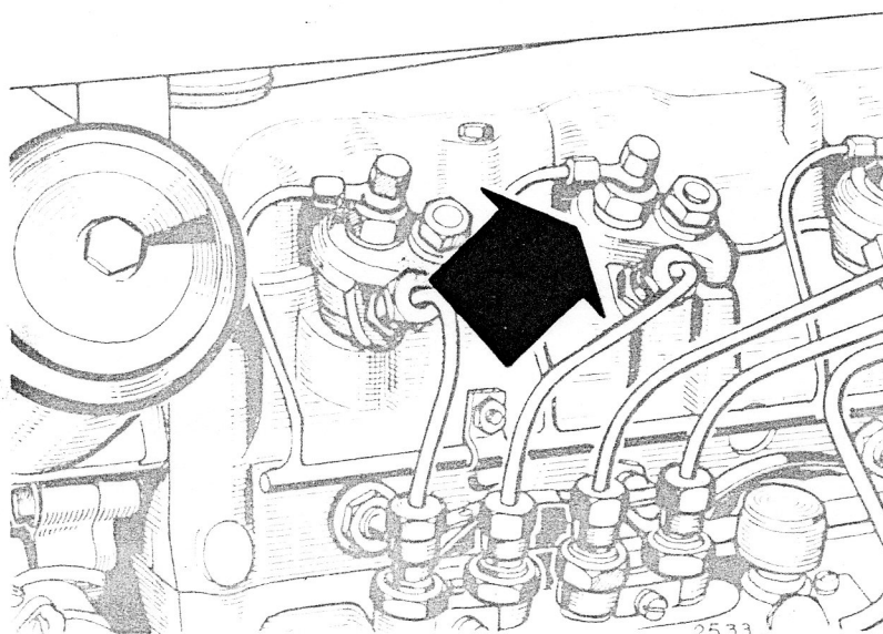
FIG. 23. — Dépose des injecteurs.
