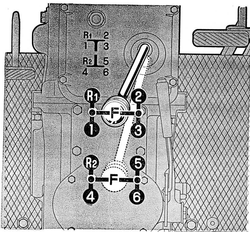
FIG. 7. — Positions du levier de changement de vitesses.
