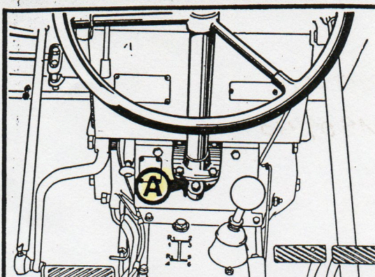
20 BOITIER DE DIRECTION - Vérifier le niveau d'huile. A= niveau et remplissage.
