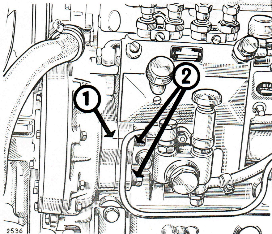
Fig. 30 B. Repères pour le calage de la pompe d'injection.
