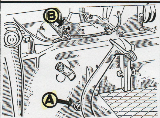
18 BOITE DE VITESSES ET TRANSMISSIONS -Vérifier le niveau d'huile. A = niveau; B= remplissage.
