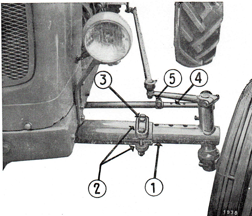
FIG. 10. — Variation de la voie avant
