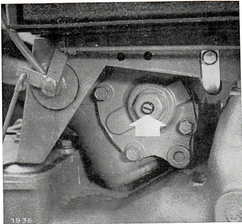
FIG. 33. — Vis de réglage de la commande de direction.
