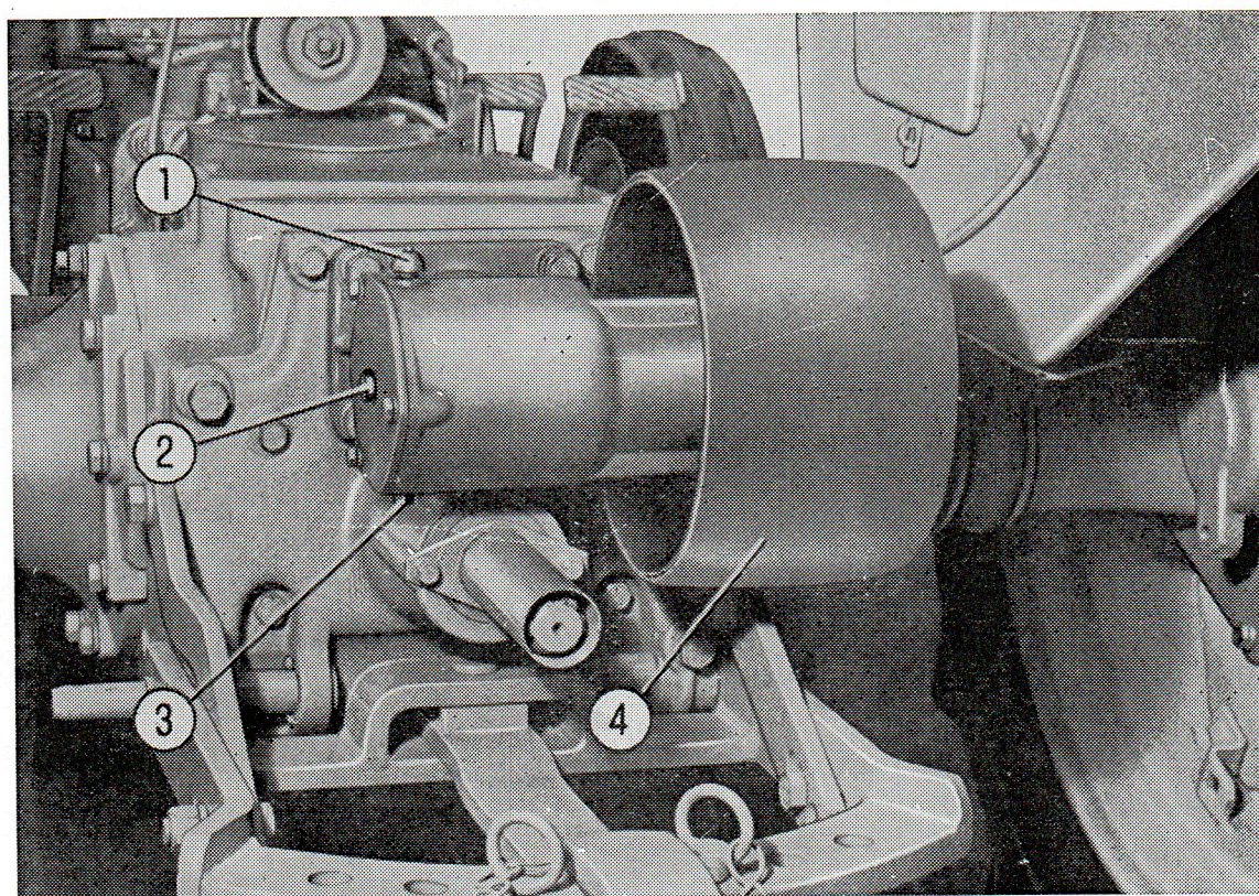
FIG. 35. — Poulie de battage.
