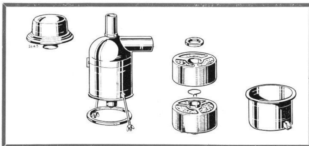
FIG. 21. — Vue des différents éléments constituant le filtre.
