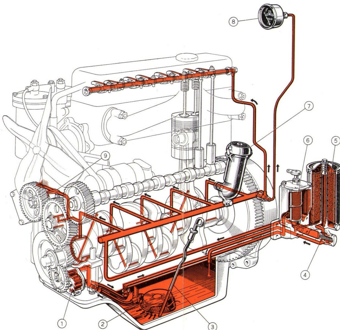
FIG. 18 ter. — Schéma de graissage du moteur.
