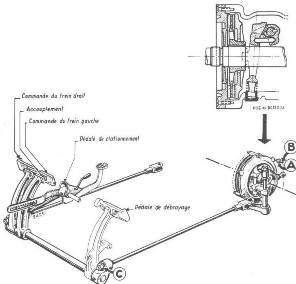
FIG. 34. — Schéma du dispositif de freinage.
