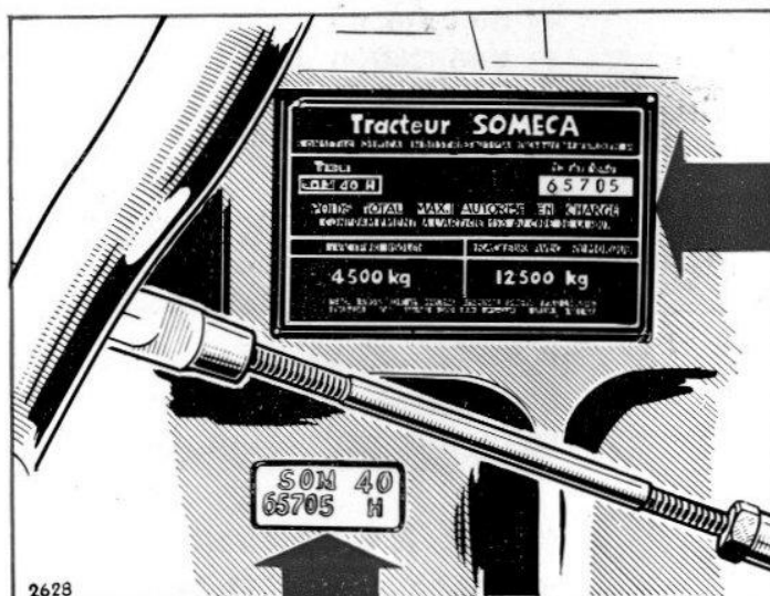
FIG. 4. — Numéro du châssis et plaque de constructeur :
