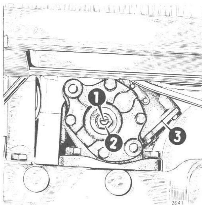
FIG. 35. — Réglage du boîtier de direction.
