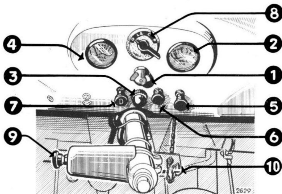
FIG. 5. - Tableau de bord
