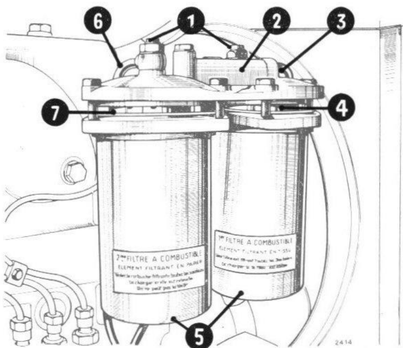
FIG. 23 - Filtres à combustible.
