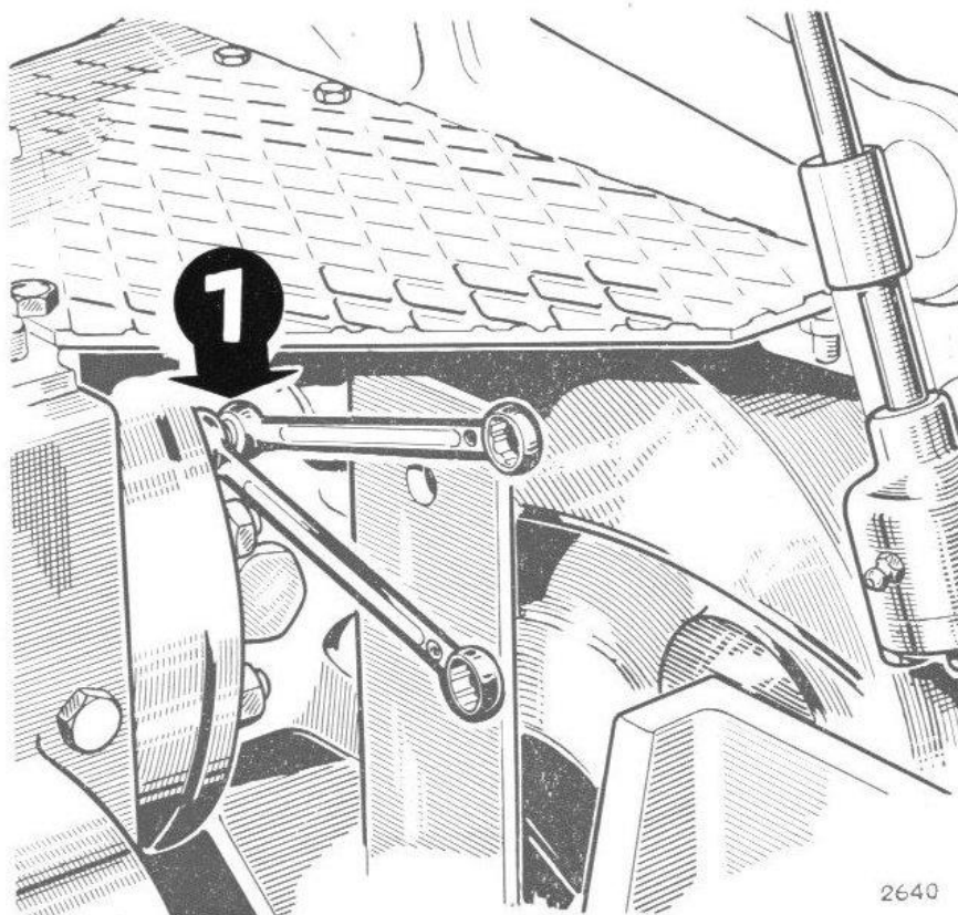
FIG. 33 - Réglage des freins.
