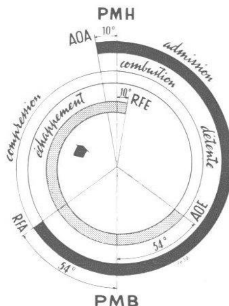
FIG. 26. - Diagramme.
