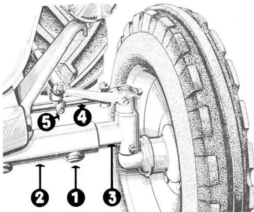
FIG. 16. — Voie avant.
