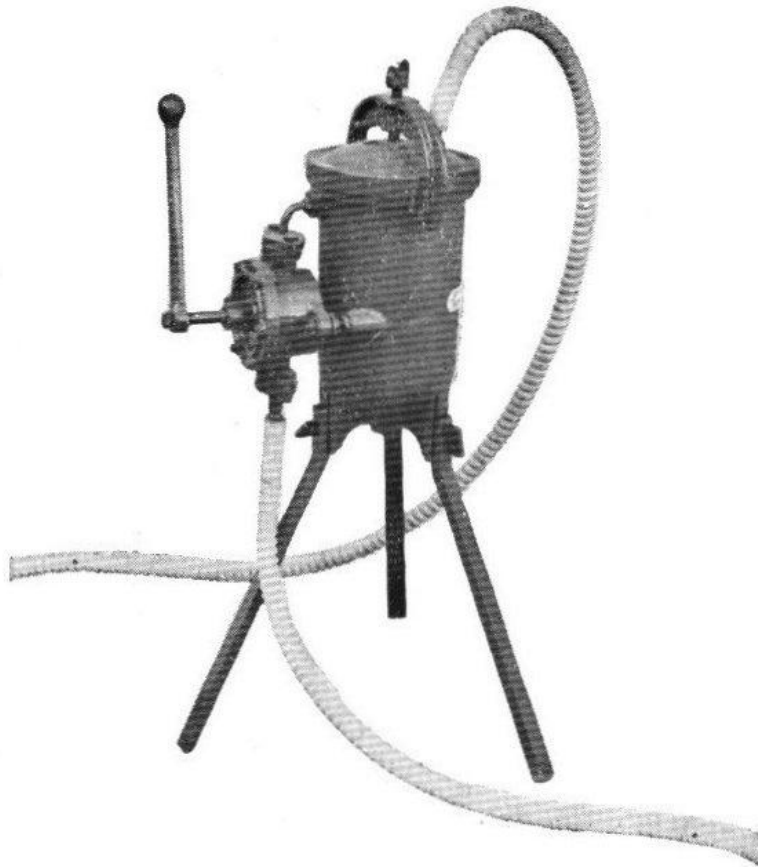
FIG. 37. – Pompe filtrante.
