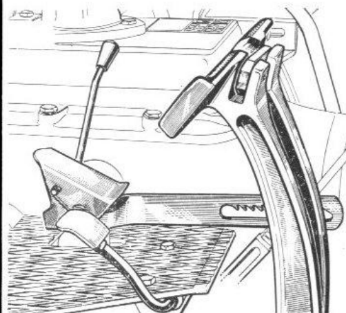
FIG. 15 — Frein de parking en position "serré."
