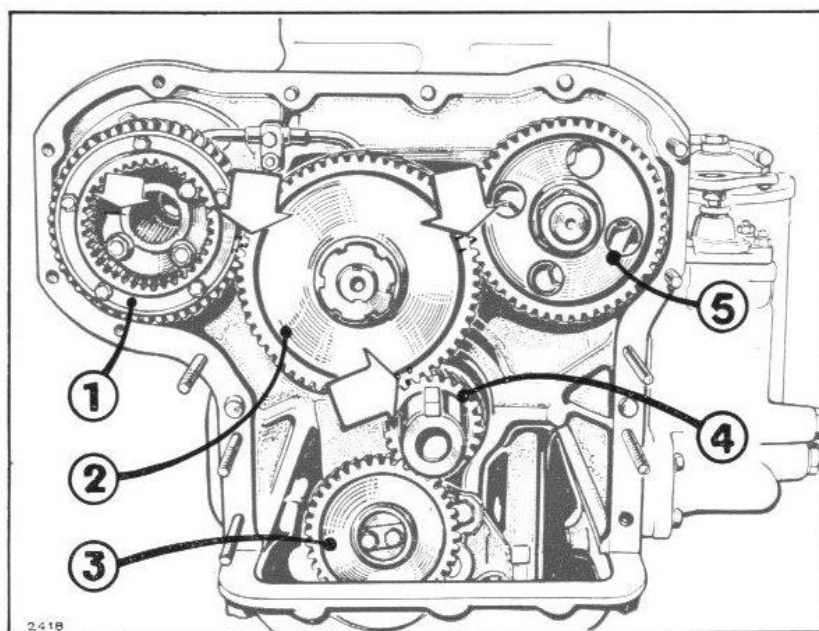
FIG. 27. – Repérage des pignons de distribution.
