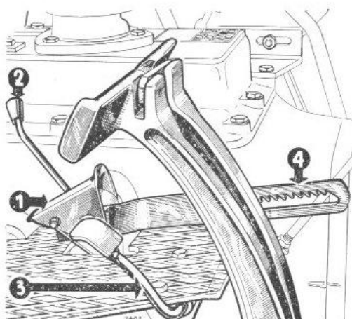
FIG. 14 — Frein de parking en position "desserré."
