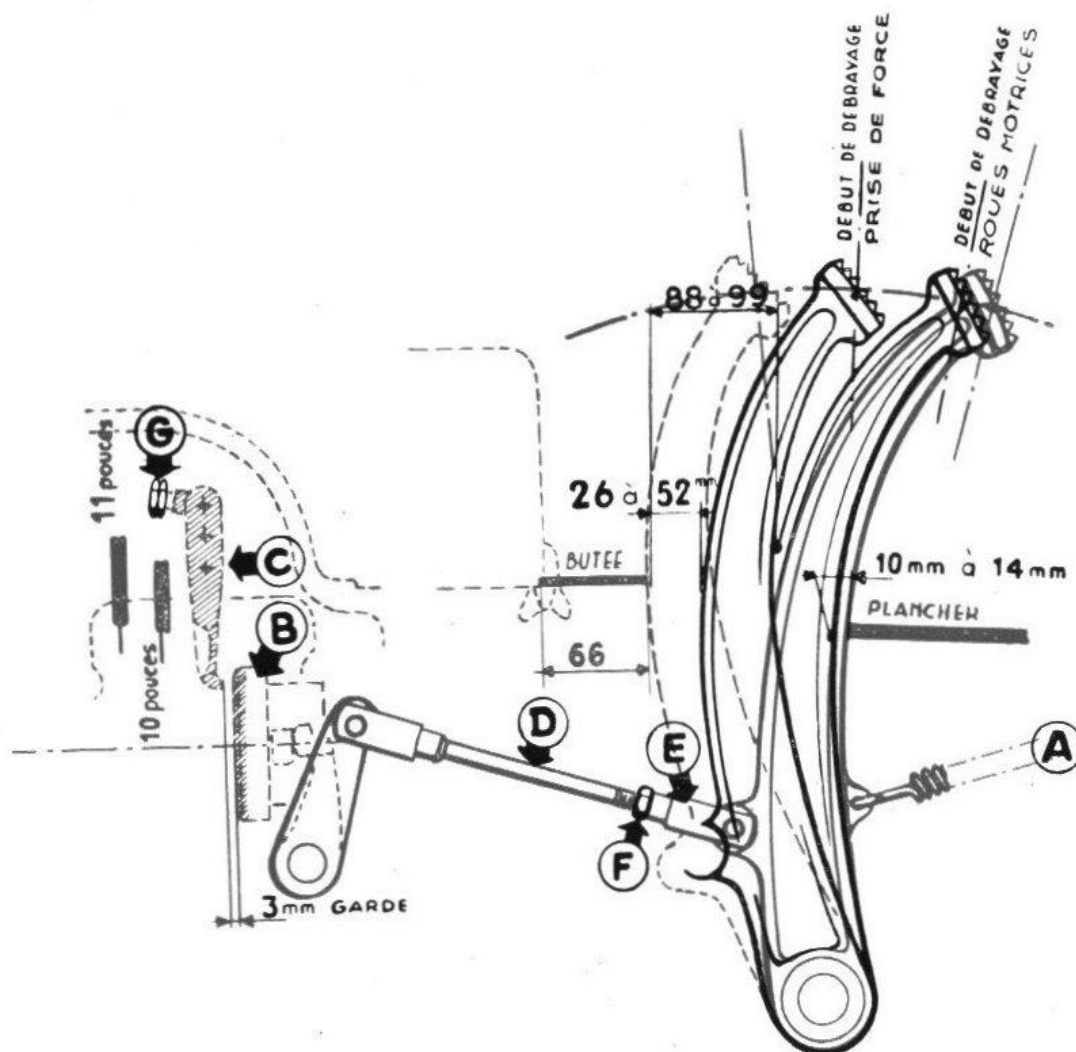
FIG. 32. - Réglage des embrayages.
