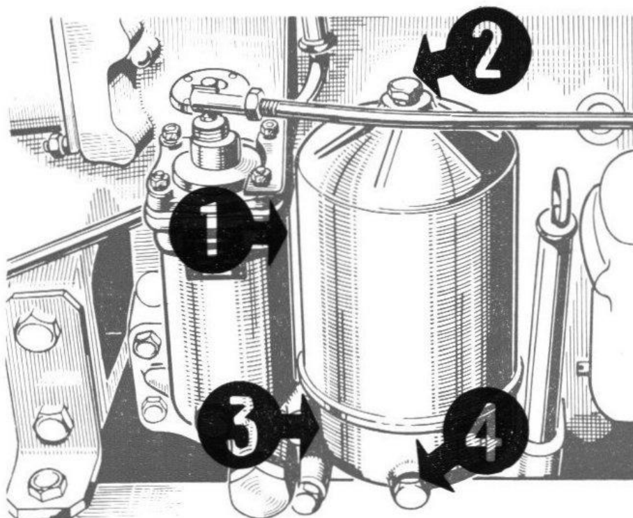
FIG. 24. – Filtre régénérateur.
