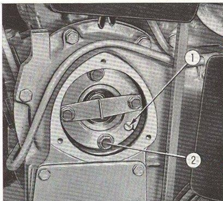
FIG. 34. — Toc d'entraînement de la pompe d'injection.
