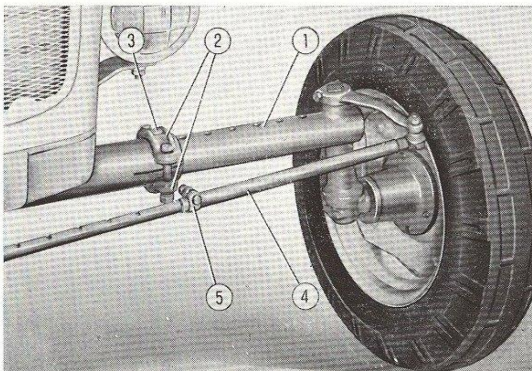
FIG. 10. — Variation de la voie avant
