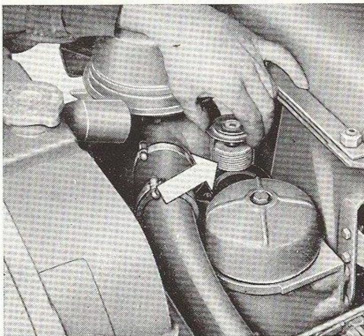
FIG. 23 — Dépose du thermostat.
