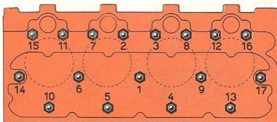
FIG. 27. Ordre de serrage des écrous de culasse.
