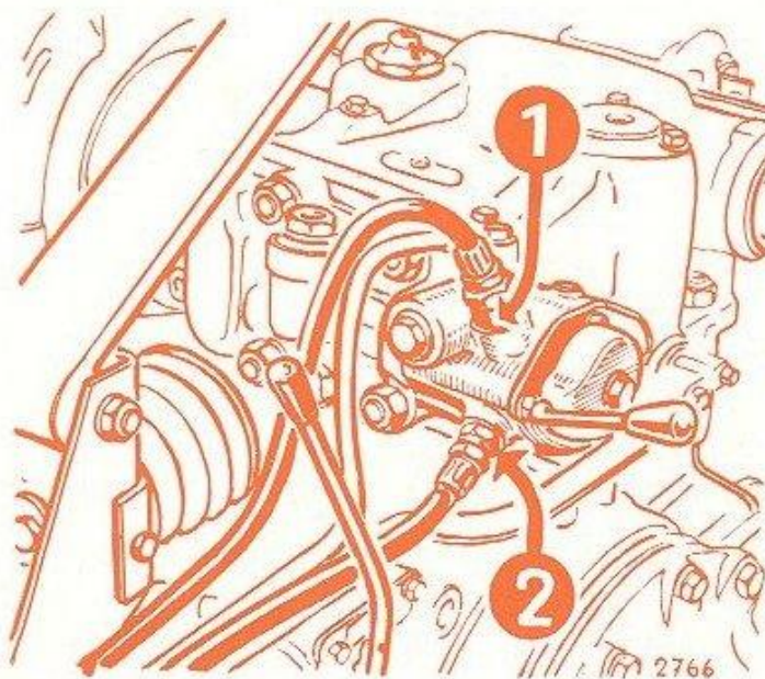
FIG. 41 — Distributeur auxiliaire équipé en double effet.
