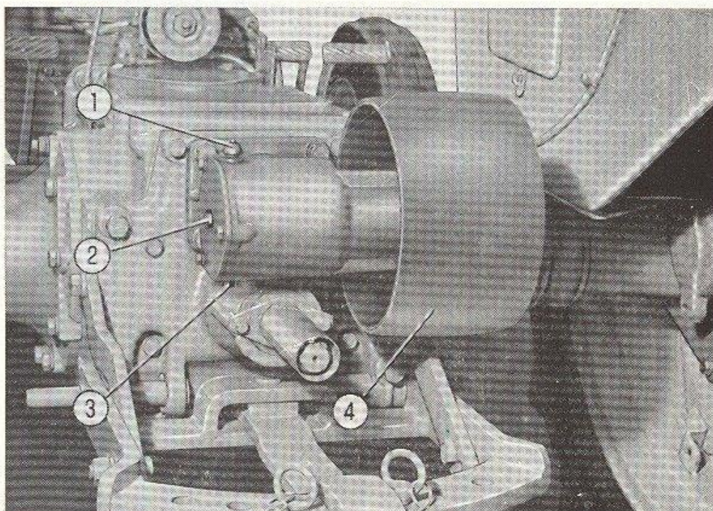
FIG. 39. — Poulie de battage.
