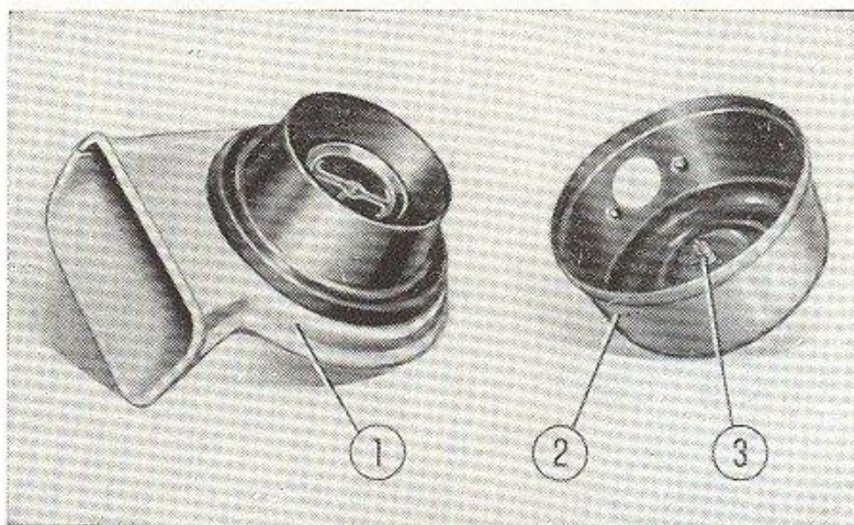
FIG. 22 — Préfiltre désassemblé
