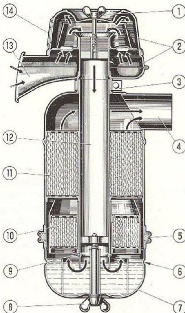
FIG. 21. — Coupe du filtre à air.
