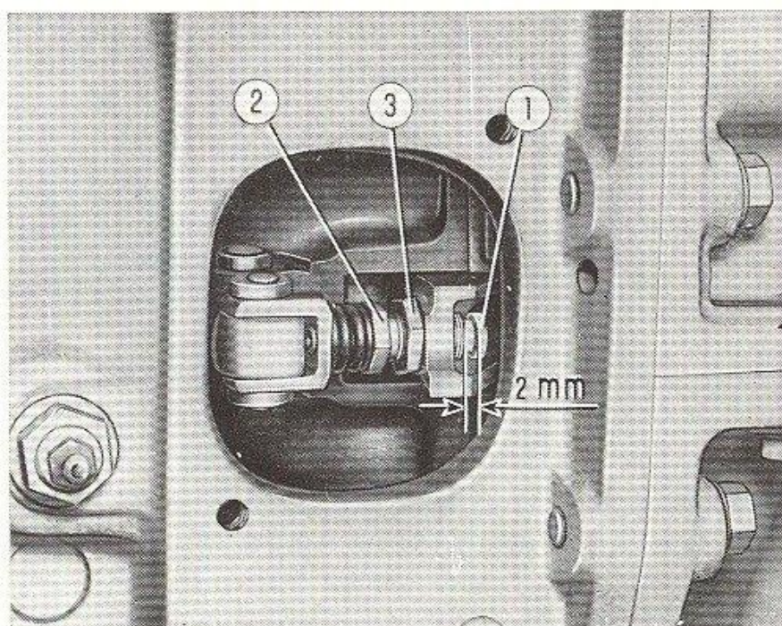
FIG. 24. — Réglage des tirants de débrayage de la prise de force.
