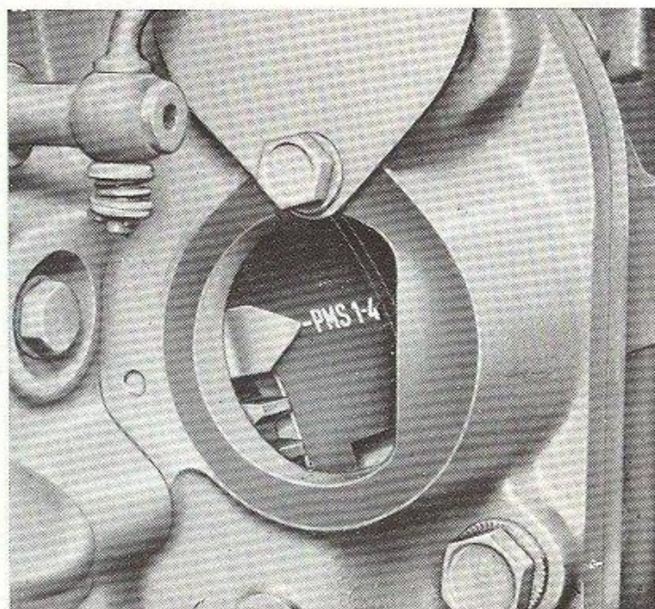
FIG. 32. — Repère sur le volant indiquant le P. M. H. des pistons N. 1 et 4.
