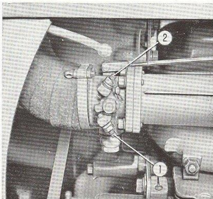
FIG. 30 — Vis de réglage du régime moteur.
