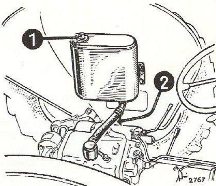
FIG. 42 — Réservoir auxiliaire.
