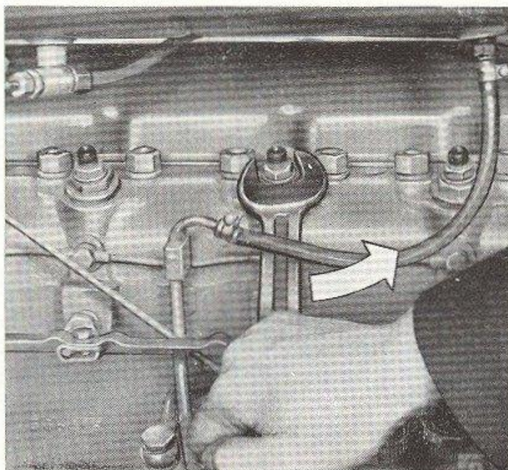
FIG. 26. — Dépose des injecteurs.
