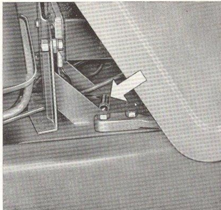
FIG. 29 — Fusible protégeant le groupe régulateur de dynamo.
