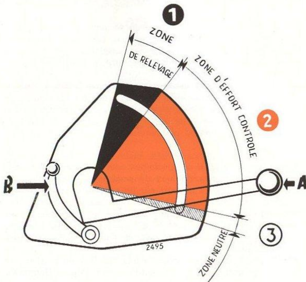
FIG. 15. — Action du levier de commande du relevage.
