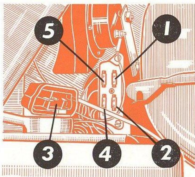
FIG. 28. — Fusibles de protection des appareils d'éclairage.
