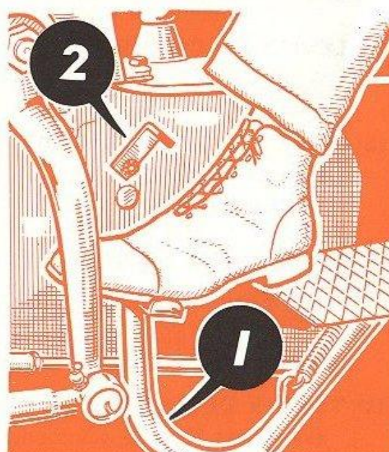
FIG. 6 B. — Pédale de débrayage (1) avec butée (2) libérant la course totale.
