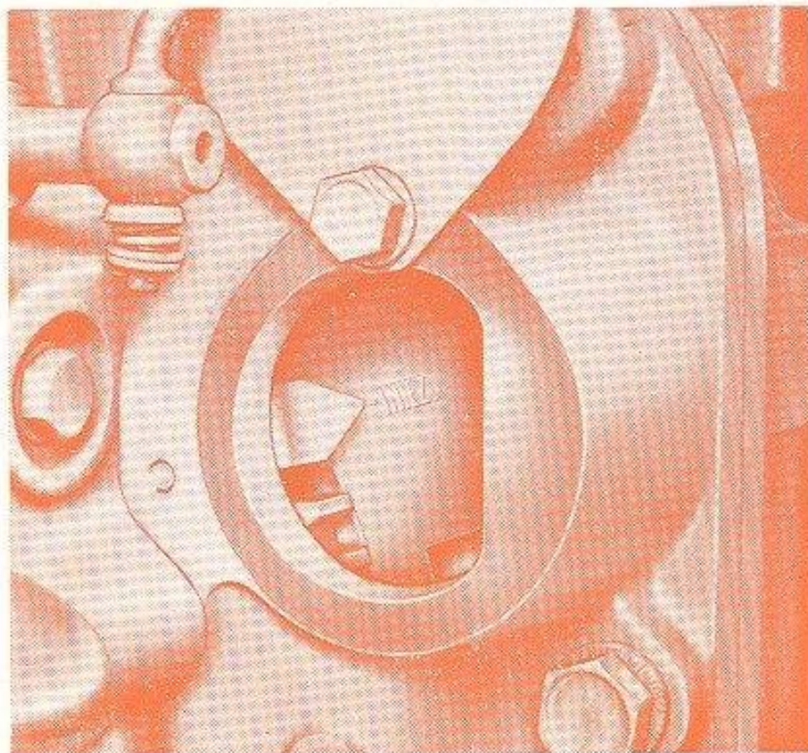
FIG. 35. — Référence sur le volant indiquant l'avance à l'injection (20° avant le P. M. H.)
