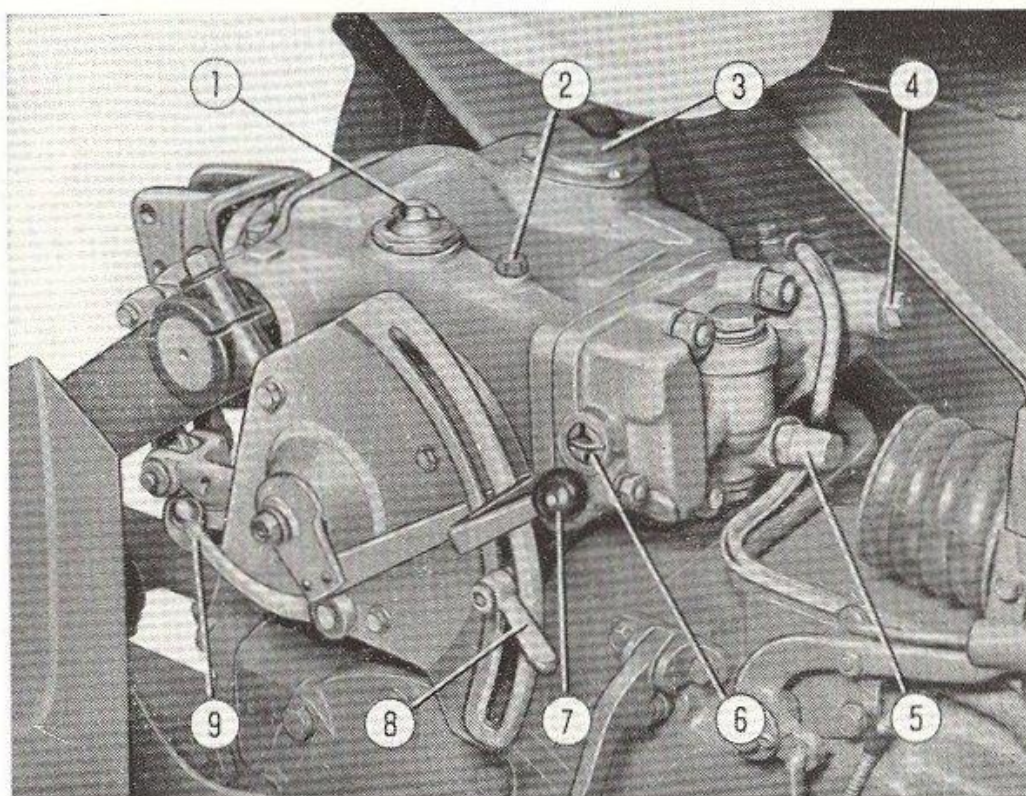
FIG. 13. — Dispositif de relevage
