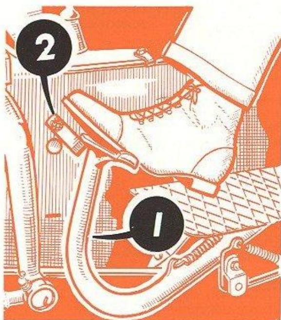
FIG. 6 A. — Pédale de débrayage (1) avec course limitée par la butée (2)
