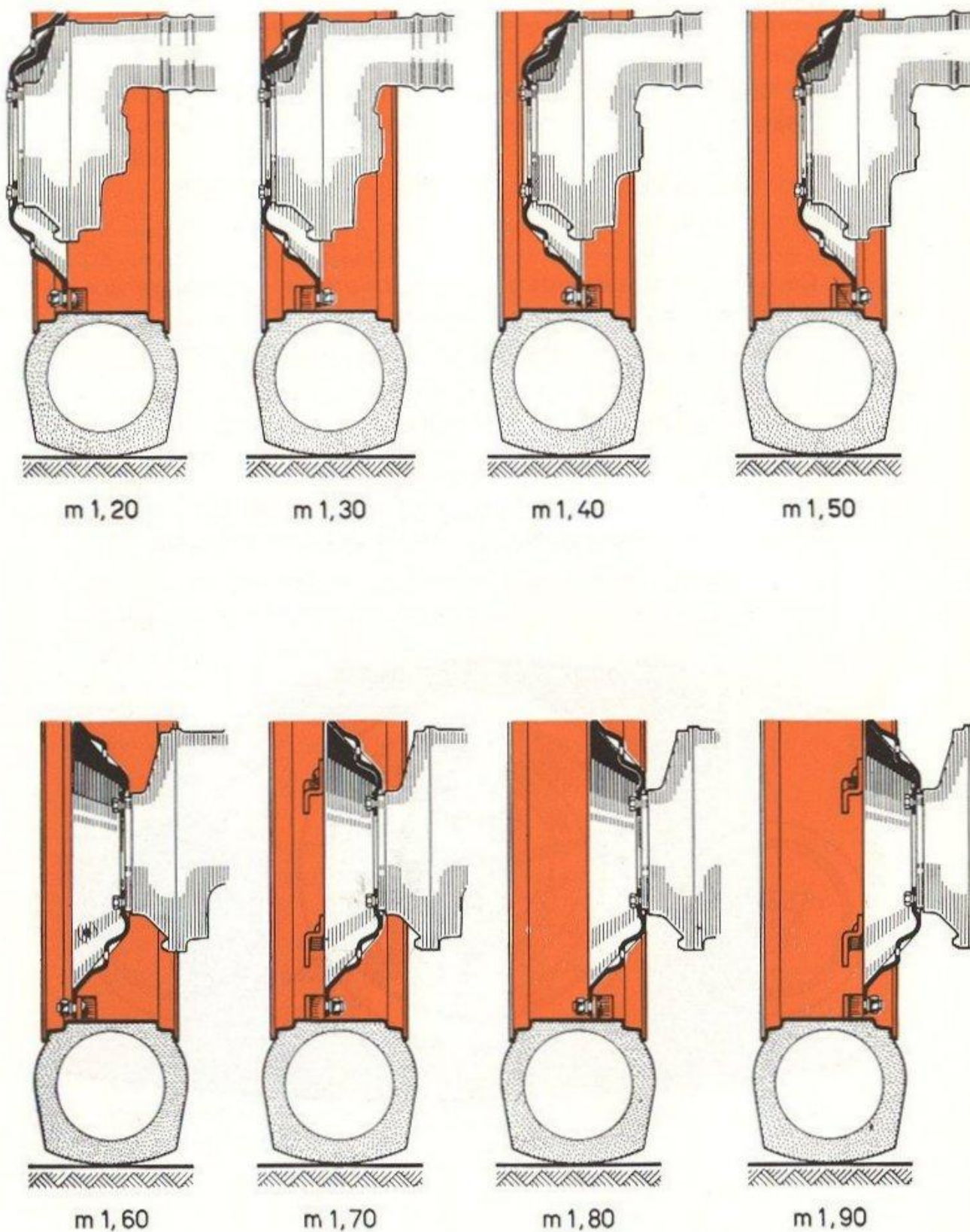
FIG. 11. — Variation de la voie arrière.
