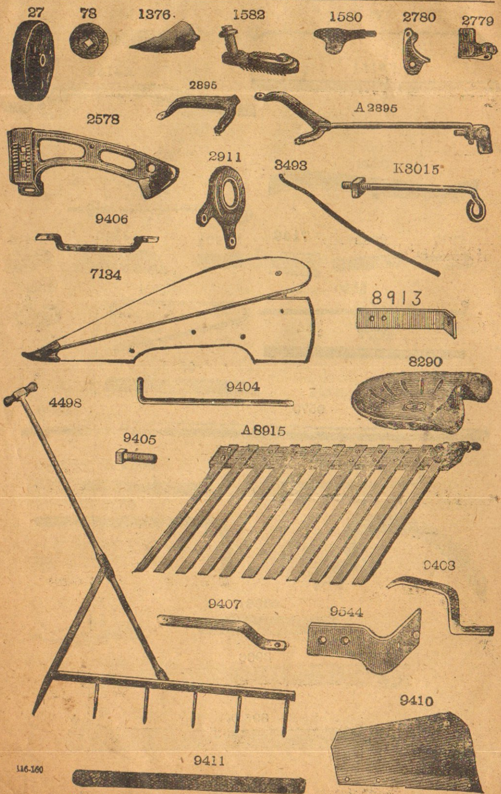
Pièces de l'appareil à moissonner avec sécateur en bois.
