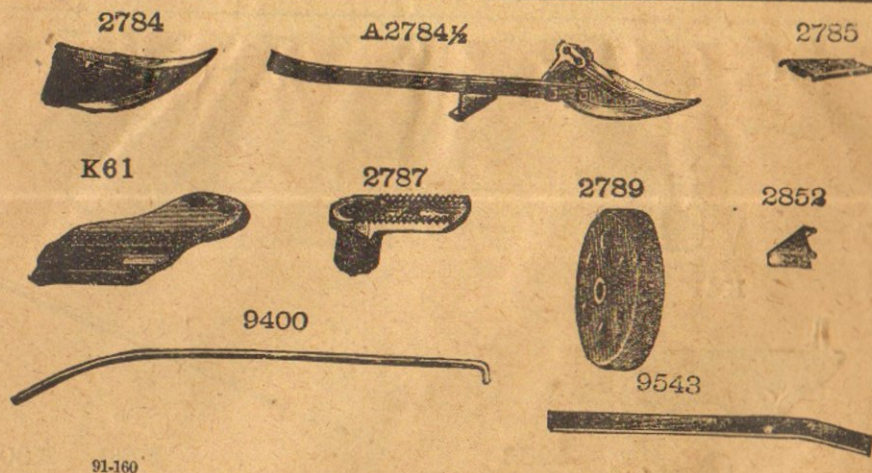
Pièces spéciales pour l'appareil à moissonner de la Faucheuse "Amiral" avec séparateur fer,
